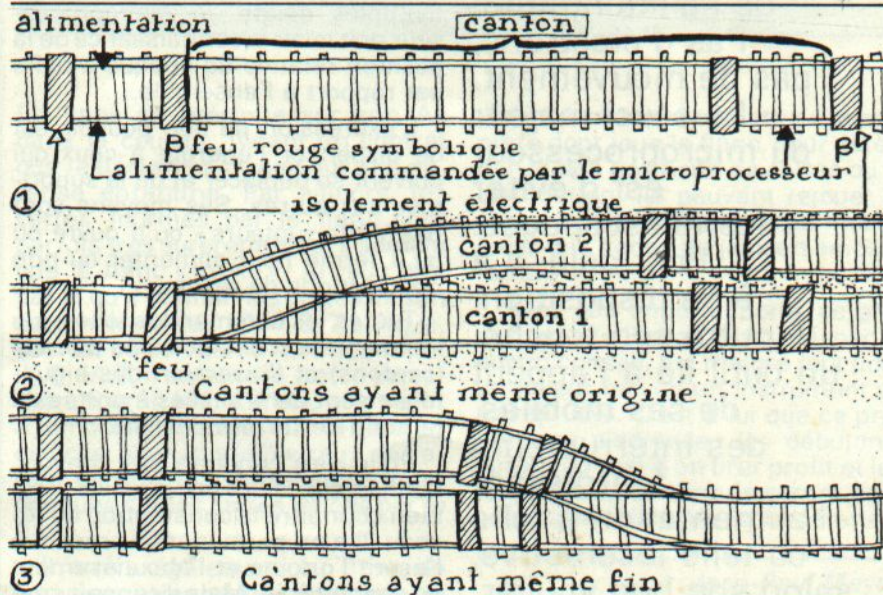
Le principe des cantons : la voie est découpée en portions appelées cantons, qui sont alimentés séparément.
